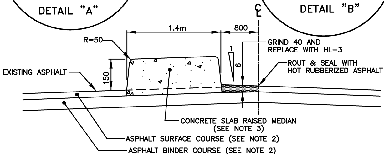
SECTION A-A
