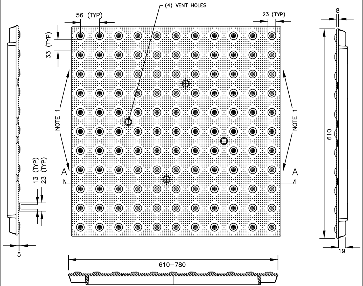
SECTION A-A
